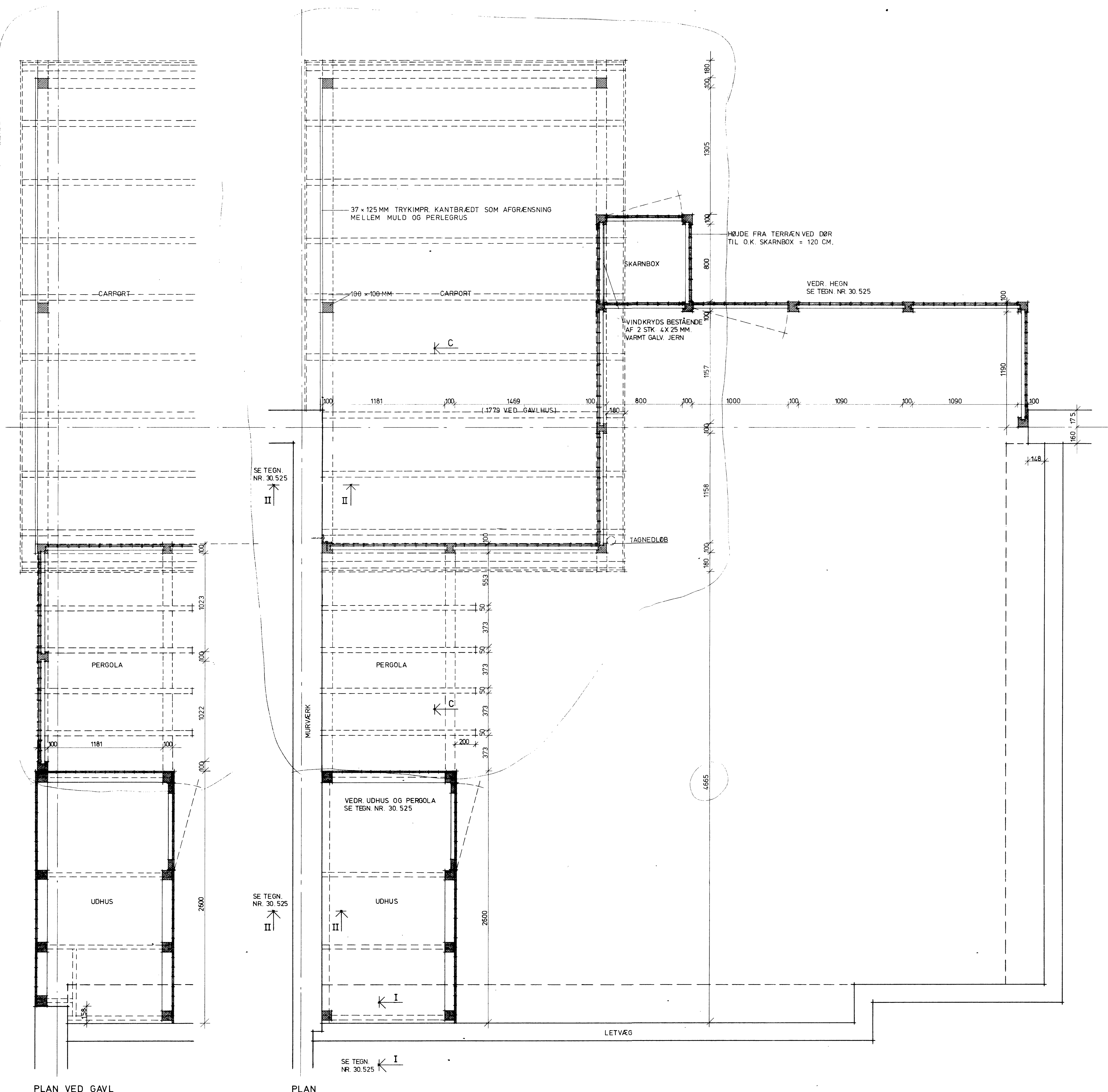
PLAN VED GAVL
