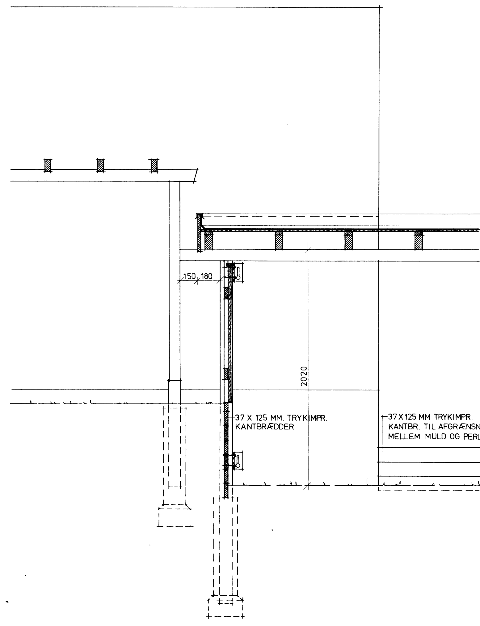
SNIT MED FORSKELLIGE TERRÆNHØJDER
